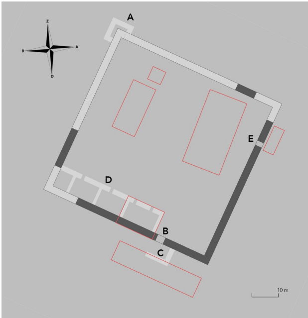
4. att. Smiltenes pils shematisks plāns. A – Z tornis B – vārtu aila DR sienā C – vārtu tornis (?) D – DR korpuss E – vārtu aila DA sienā Gundara Kalniņa zīmējums, 2023
