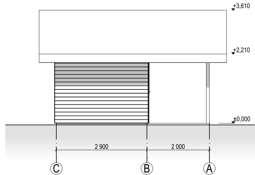
Fasāde asīs C-A
