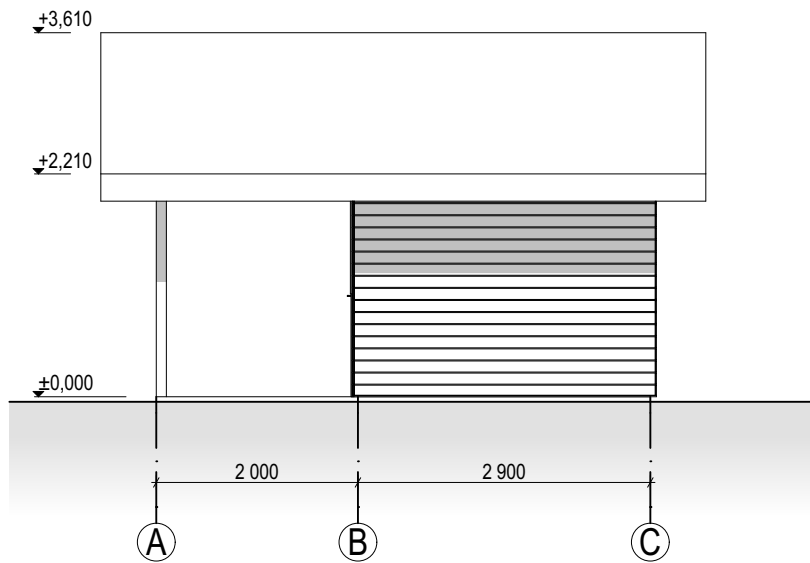
Fasāde asīs A-C
