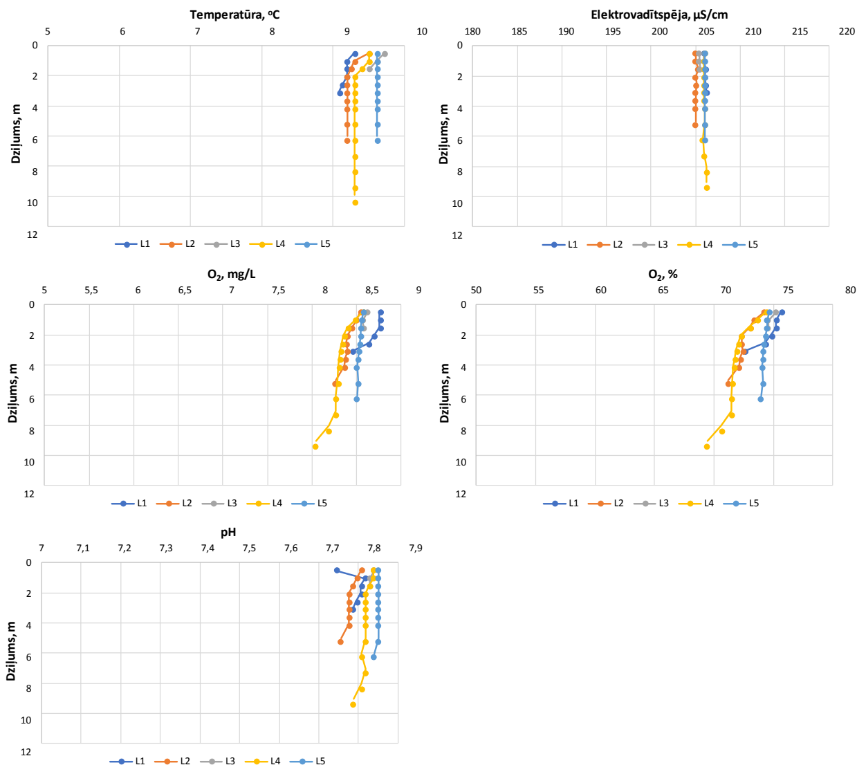
5.2.3. attēls. Fizikāli ķīmisko parametru stratifikācija Lidoles ezerā 16.10.2019.
